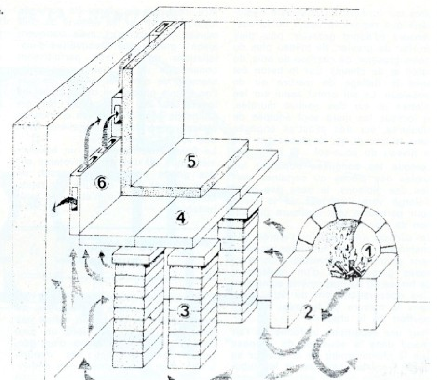
Schéma de principe d'un hypocauste. 1. Foyer. 2. Conduit de chaleur. 3. Pilette d'hypocauste. 4. Suspensura (brique ou pierre). 5. Sol bétonné. 6. Tubulures murales (tubuli). Dessin d'après Filtzinger.
